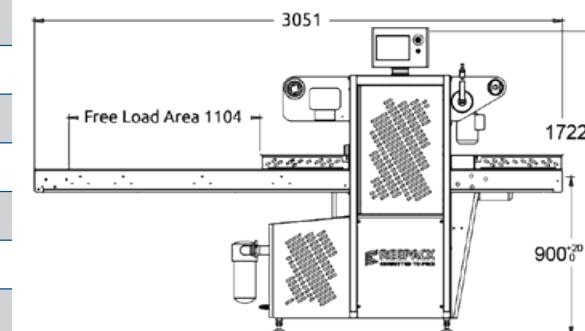
Πλάγια όψη
